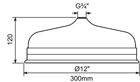
12" Easy clean shower rose 12 Zoll Easy Clean Kopfbrause Pomme de douche ronde, entretien facile, de 300 mm Rociador de ducha redondo de fácil limpieza de 300 mm Soffione easy clean da 12"
