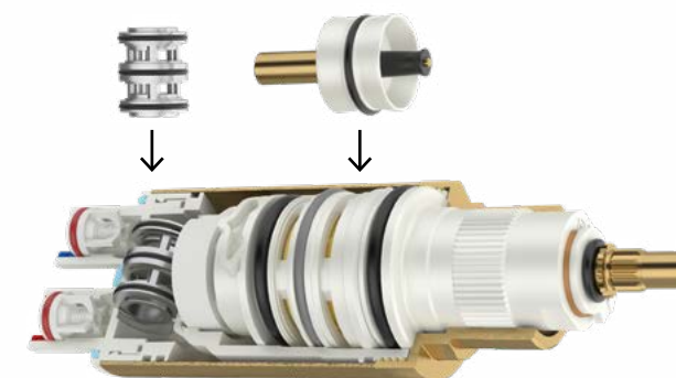
KARTUSCHE / CARTUCCIA
